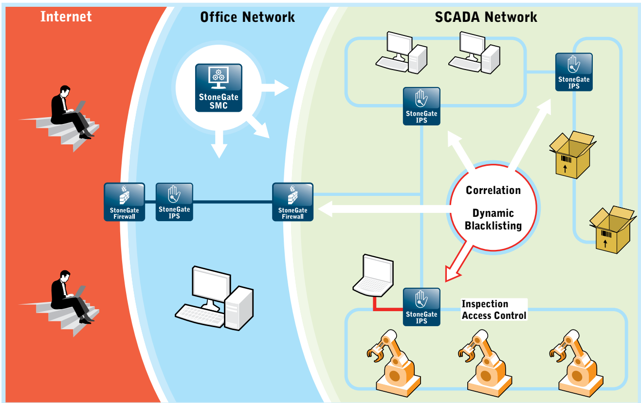
Die Stonegate IPS Transparent Access Controll Lösung im Unternehmensnetzwerk
